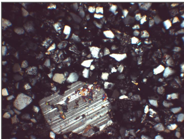
Fig.2. Plagioklas med sekundärmineraliseringar i en finkornigare grundmassa av huvudsakligen kvarts samt fältspater, 10x XPL.
