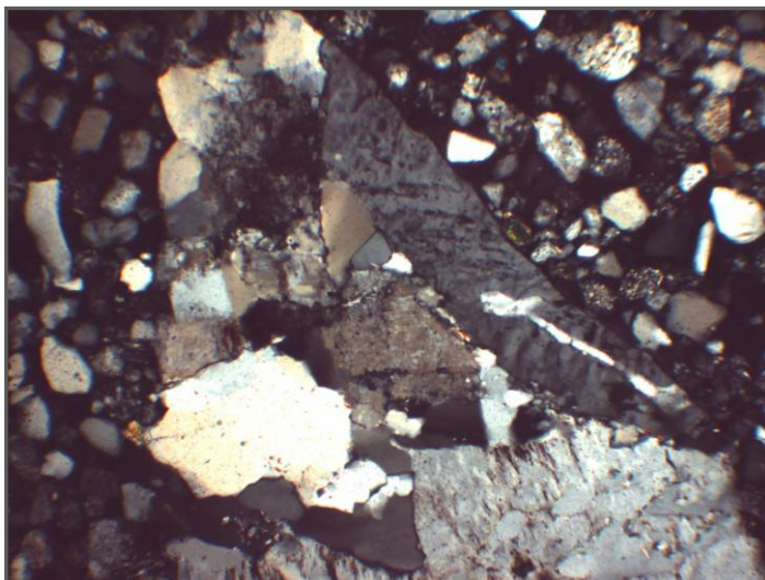
Fig.3. Ca 1,6 mm brett aggregat av fältspater samt kvarts, 10x XPL.
